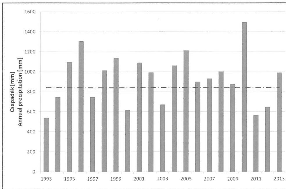
7. ábra: Éves csapadékok 1993 és 2013 között (jelölve az átlag csapadék: 840 mm) Fig. 7.: Annual precipitation 1993-2013 (marked the average precipitation: 840 mm)
