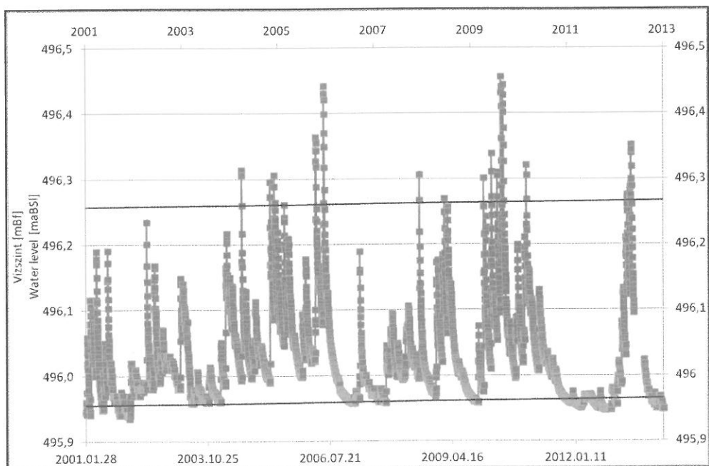
12. ábra: Garadna-forrás vízszintadatai 2001 és 2013 között, jelölve a éves maximumok és minimumok trendje Fig. 12.: Water level in Szinva spring between 2001 and 2013 and the characteristic trend line of yearly maximums and minimums
