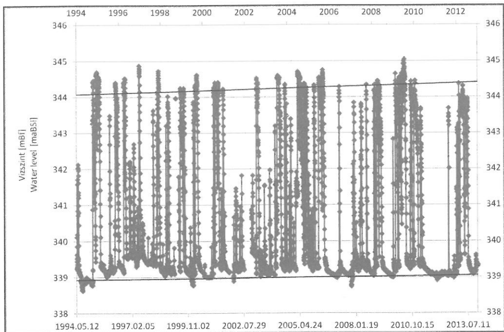
11. ábra: Szinva-forrás vízszintadatai 1994 és 2013 között, jelölve a éves maximumok és minimumok trendje Fig. 11.: Water level in Szinva spring between 1994 and 2013 and the characteristic trend line of yearly maximums and minimums
