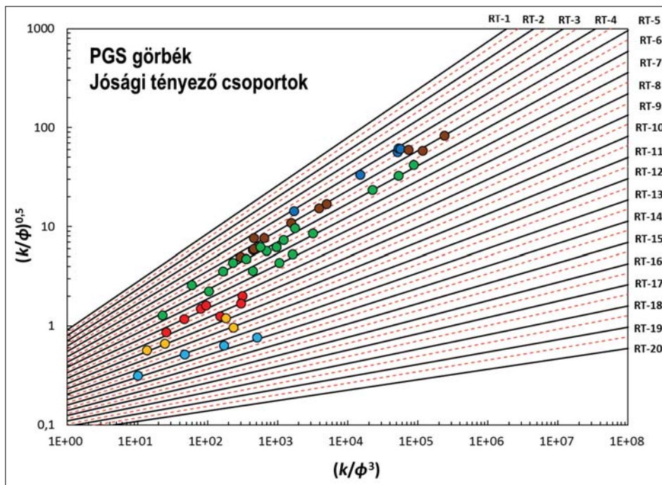
3. ábra | Homokkőminták osztályozása a jósági tényező alapján alapján a PGS módszer felhasználásával
