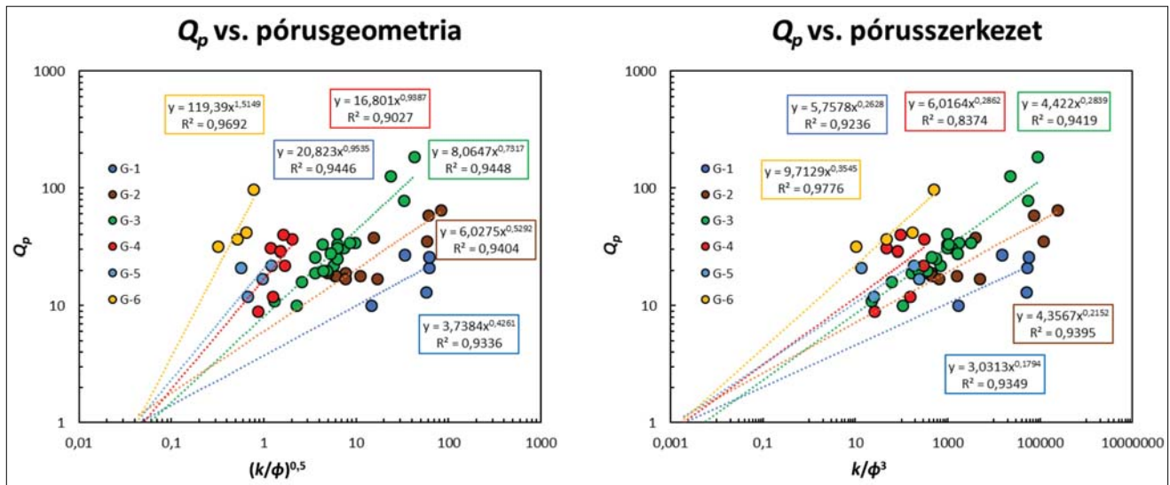
4. ábra | A jósági tényező kapcsolata a pórusgeometriával és pórusstruktúrával a PGS módszerrel való csoportosítás alapján
